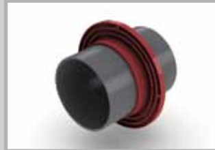
Futterrohr aus Kunststoff Mit Mittelflansch. Innendurchmesser: 60–500 mm
